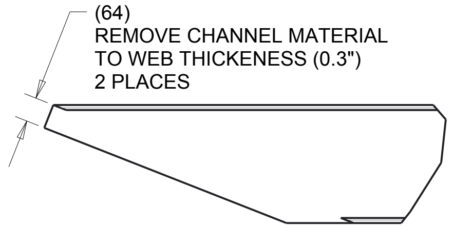
DETAIL A SCALE 0.100
